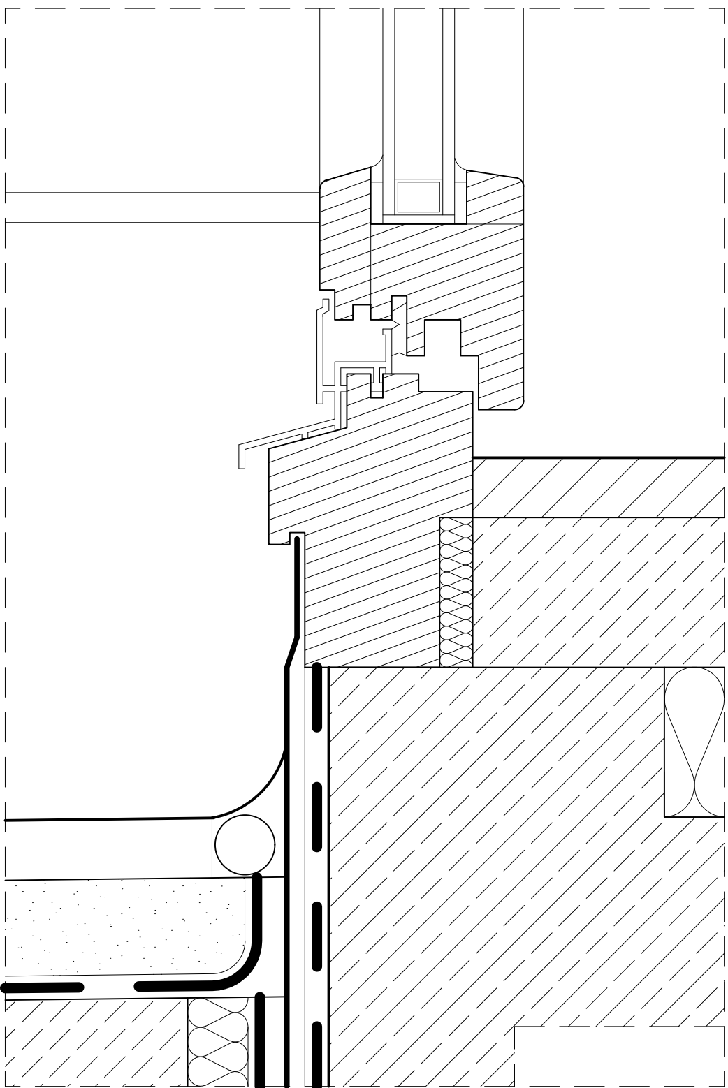
Дерев'яна рама
